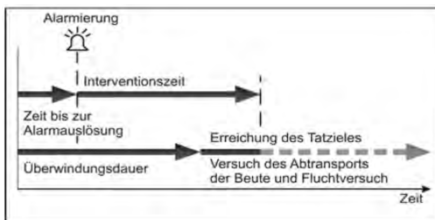
Bild 5.02 Verbesserter Ablauf mit aufeinander abgestimmtem Zusammenwirken von mechanischen und elektronischen Sicherungseinrichtungen
