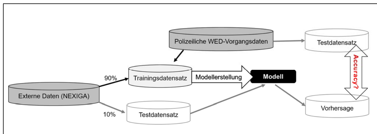
Abbildung 26: Datenaufteilung für Modellerstellung und Validierung mittels Accuracy Index
