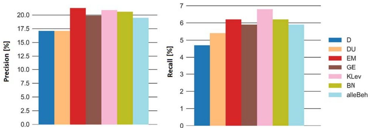
Abbildung 38: RZC-Score: Vergleich (Precision und Recall) für die Top2 % der Prognosegebiete nach Pilotbehörden
