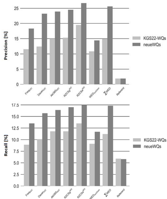
Abbildung 40: RZC-Score: Vergleich für Wohnquartiere
