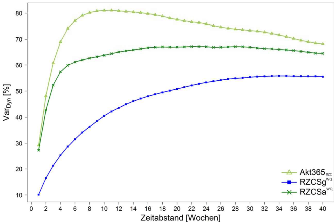
Abbildung 41: RZC-Score: Vergleich Zeitliche Dynamik der WED-Prognosen in Wochenabständen
