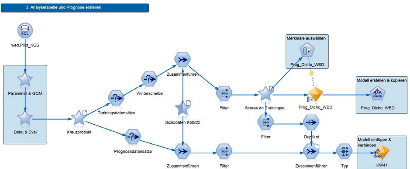
Abbildung 16: Beispiel-Stream: Prognoseerstellung, 1. Teil
