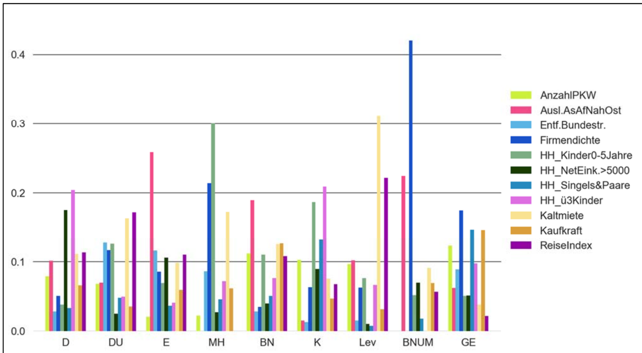
Abbildung 31: Einflussstärke der soziostrukturellen Daten beim Random-Forest-Modell nach Bezirken
