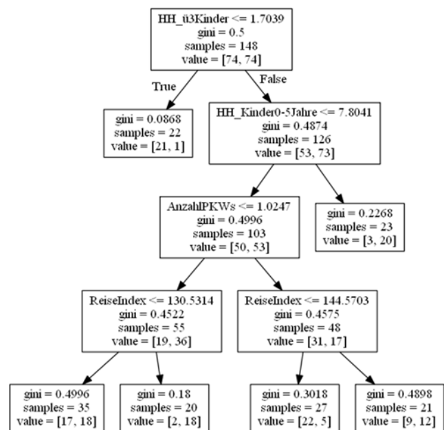
Abbildung 25: Beispiel-CART-Klassifizierungsbaum
